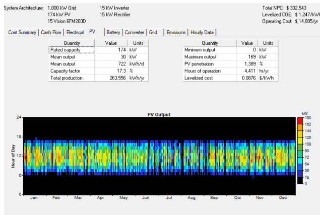
Fig. 4.5 PV output
